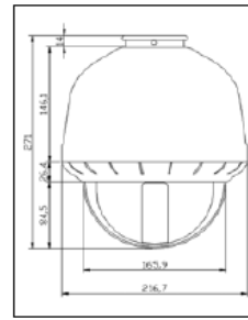
Dimension :mm
